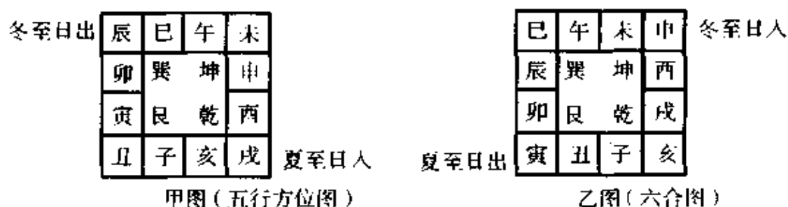
图 2-3 太阳周年视运动方图
