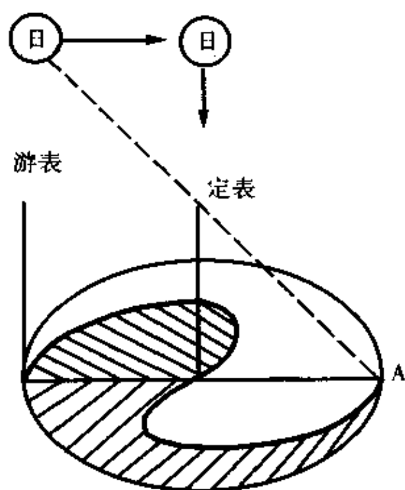
图 4-16 秋冬二季太阳视运动投影图
