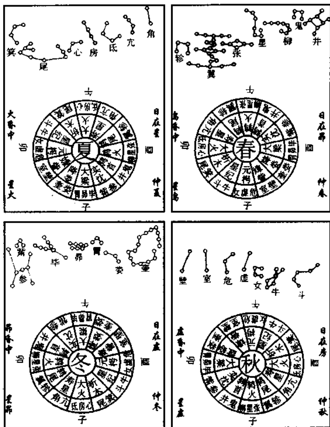
图 2-15 《尧典》四仲中星图
