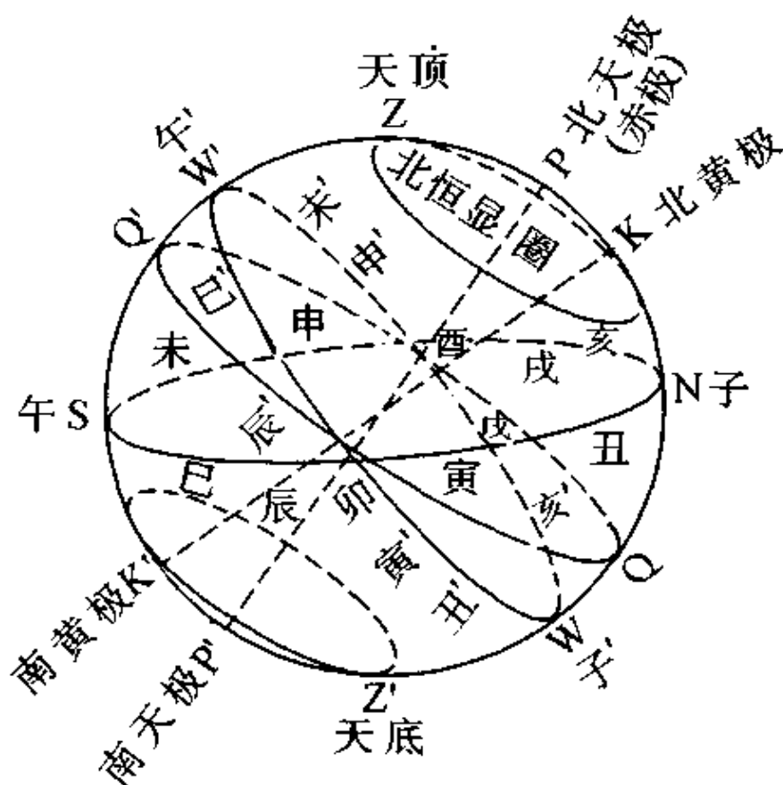
图 2-5 地平、黄赤坐标图
