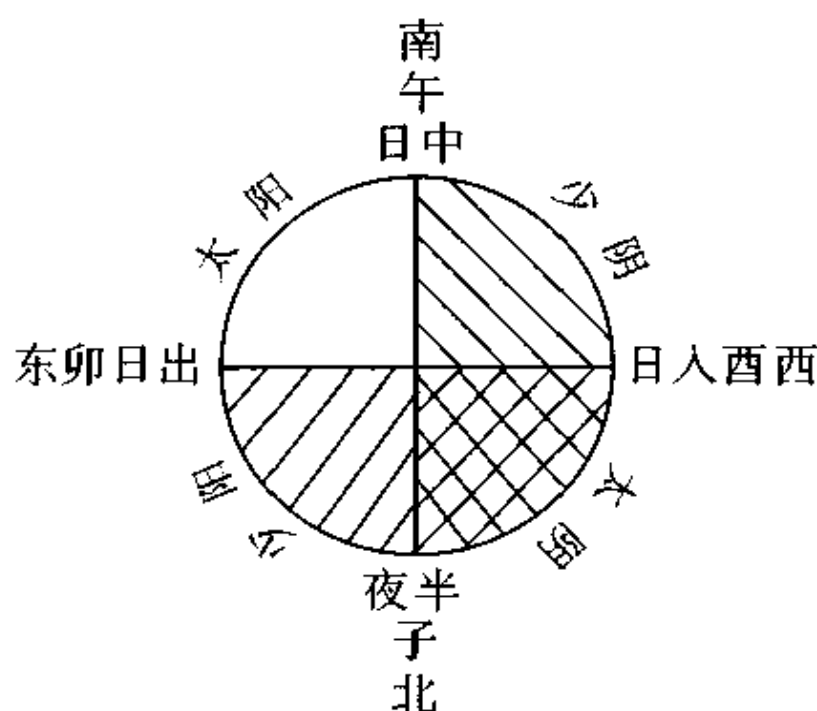
图 2-1 太阳周日视运行图（即四象图）
