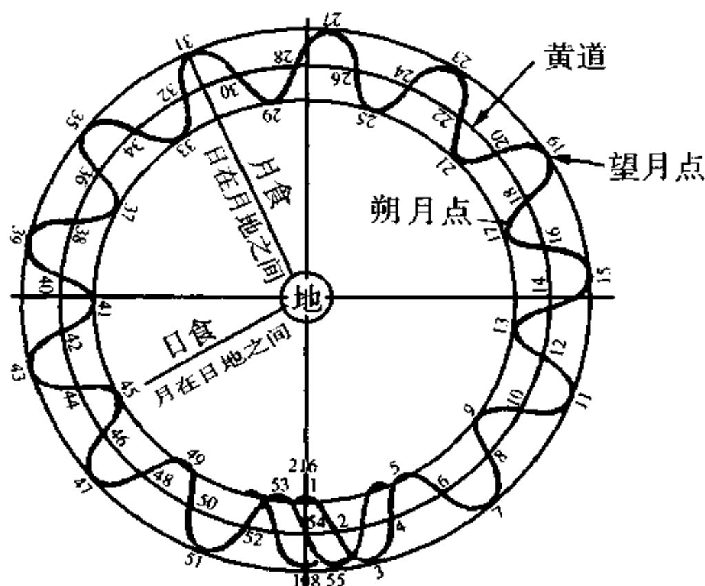
图 2-9 月亮运行轨迹在黄道面上的投影
