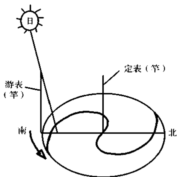
图 4-15 立竿测影示意图
