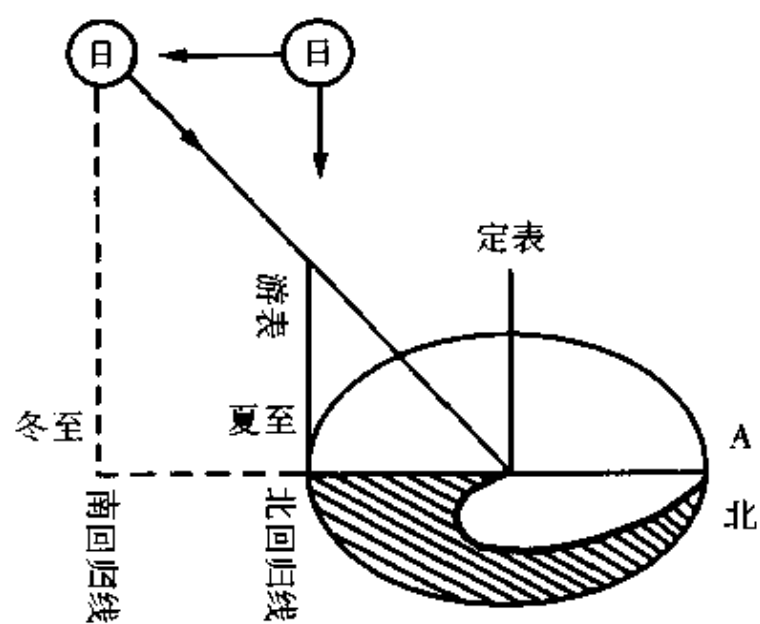
图 4-16 秋冬二季太阳视运动投影图
